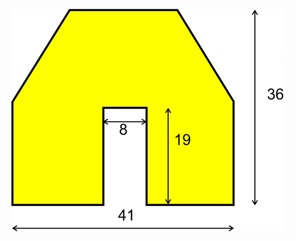
Przekrój i wymiary profilu (mm):
